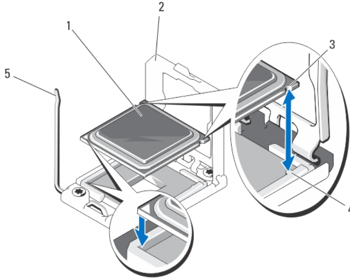
그림 14. 프로세서 분리 및 설치
