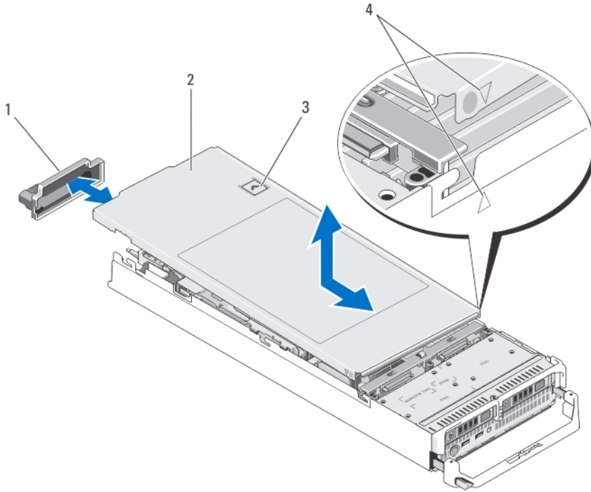
그림 4. 블레이드 열기 및 닫기
