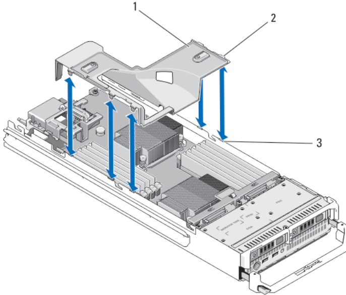
그림 6. 냉각 덮개 분리 및 설치
