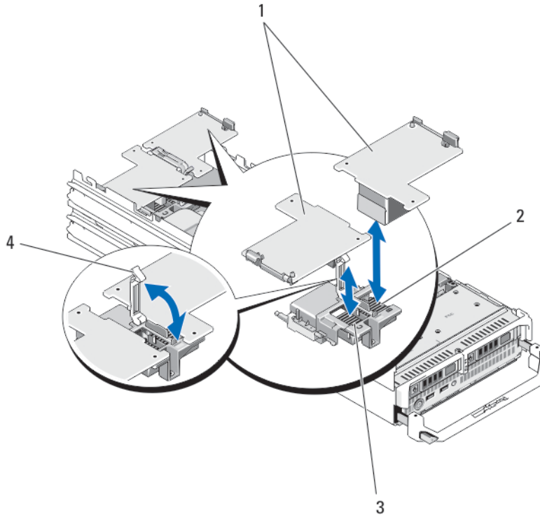
그림 9. 메자닌 카드 분리 및 설치
