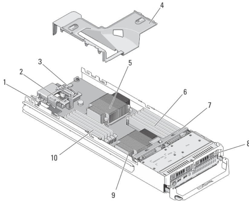
그림 5. 블레이드 내부
