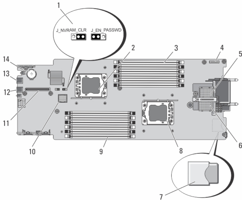
그림 21. 시스템 보드 커넥터
