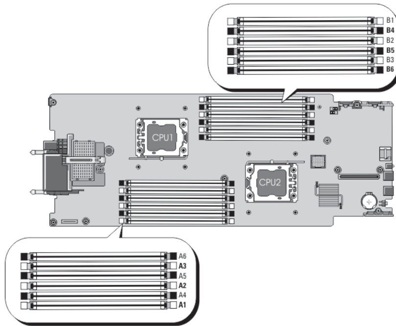
그림 7. 메모리 소켓 위치
