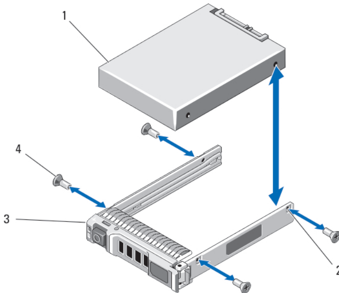
그림 16. 하드 드라이브/SSD 캐리어에서 하드 드라이브/SSD 분리 및 설치
