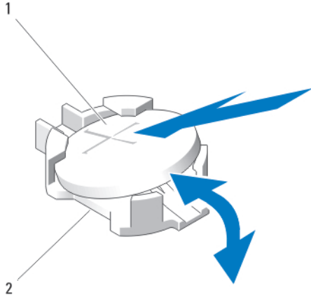
그림 19. NVRAM 백업 전지 장착
