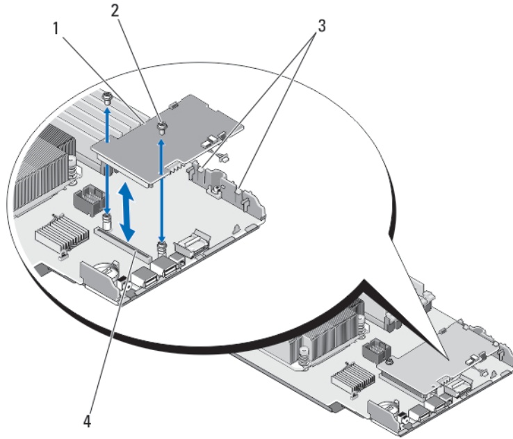
그림 20. 저장소 컨트롤러 카드 분리 및 설치
