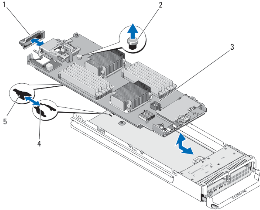
그림 18. 시스템 보드 분리 및 설치
