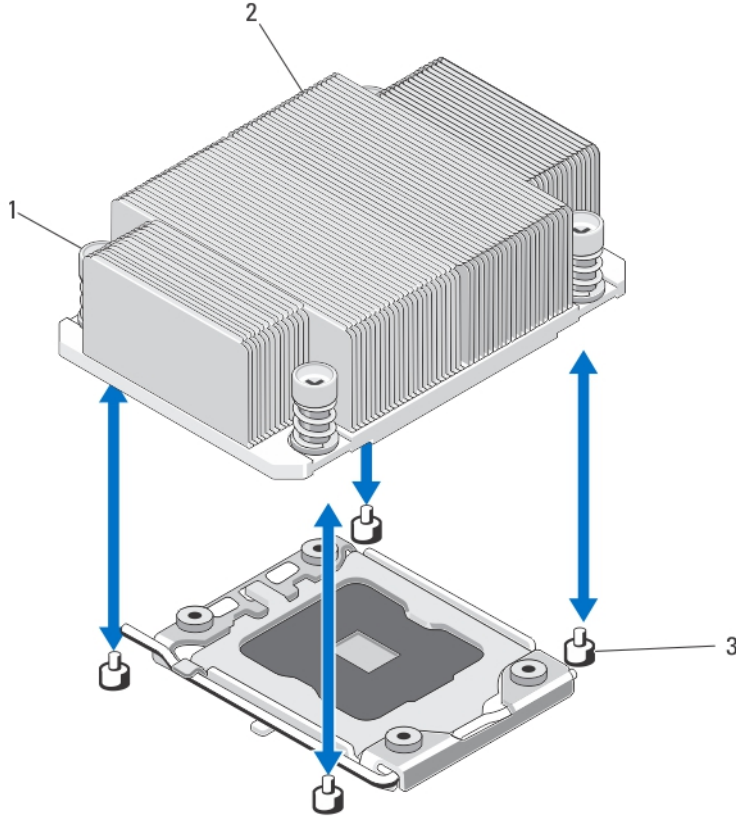
그림 13. 방열판 분리 및 설치
