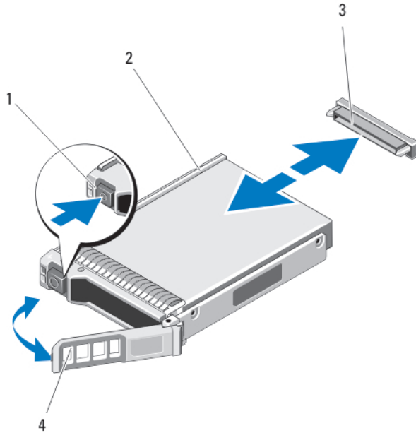
그림 15. 하드 드라이브/SSD 분리 및 설치
