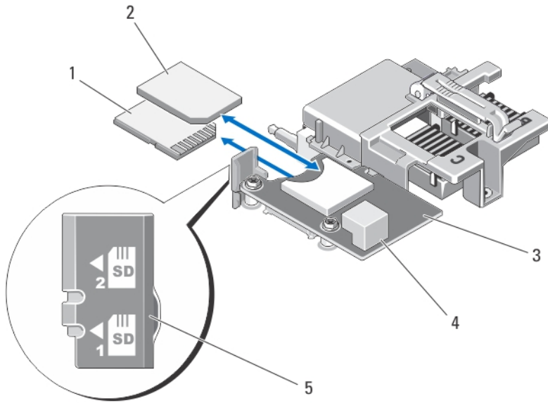
그림 10. SD 카드 장착
